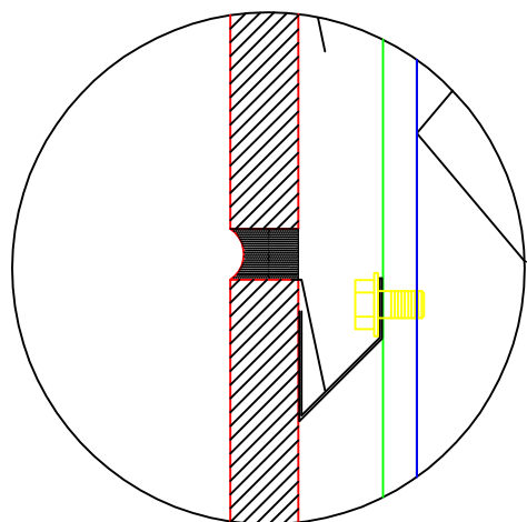
HORIZONTELL RÖRELSESKARV h=15 mm ELASTISK MASSA ELEMENTETS STOMME FIXERAS INTE MED SKRUVAR
