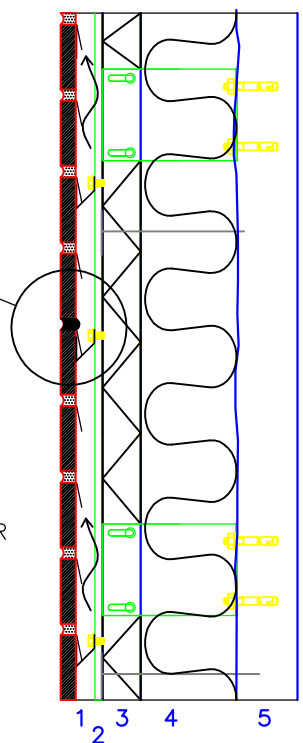
HORIZONTELL RÖRELSESKARV h=15 mm ELASTISK MASSA ELEMENTETS STOMME FIXERAS INTE MED SKRUVAR
